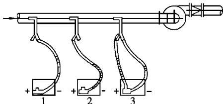
1 - 全负压;2 - 静负压;3 - 动压
