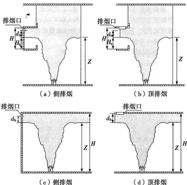
图 19 排烟口设置位置参考图
