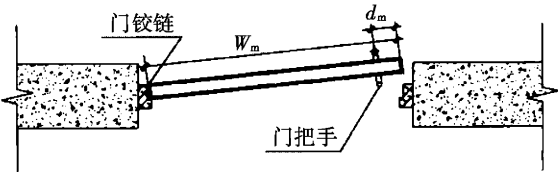
图 5 防火门开启示意图
