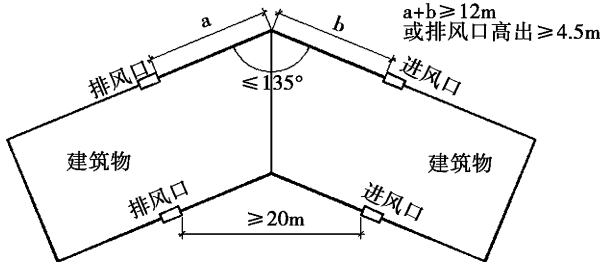
图 4 进风口与排烟口位置示意图
