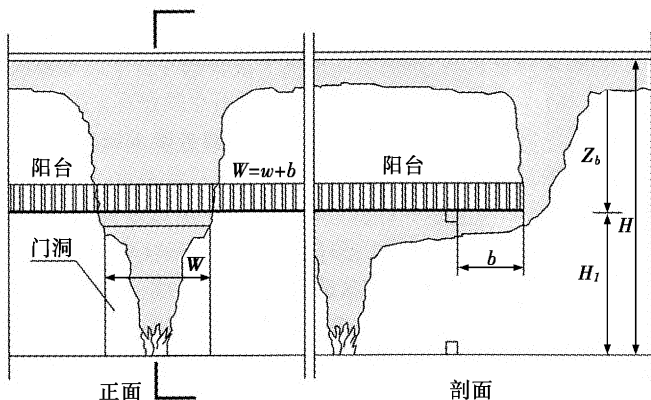
图 14 阳台溢出型烟羽流
