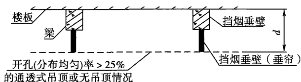
图 6 无吊顶或设置开孔(均匀分布)率大于 25% 的通透式吊顶
