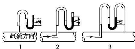
1 - 静压;2 - 全压;3 - 动压
