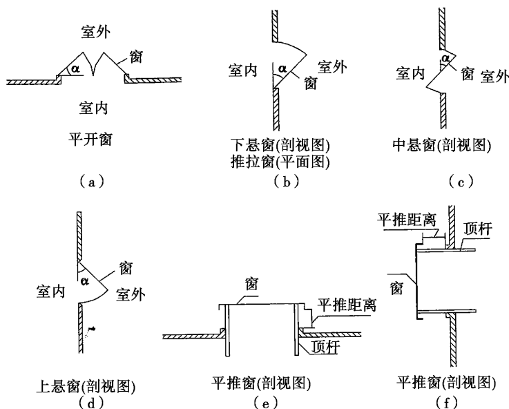
图9 可开启外窗示意图
