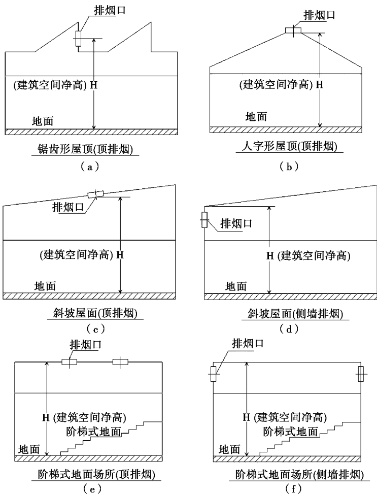
图 12 空间净高示意图
