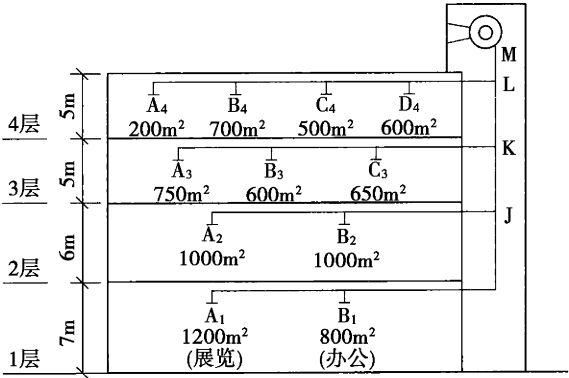
图 10 排烟系统示意图
