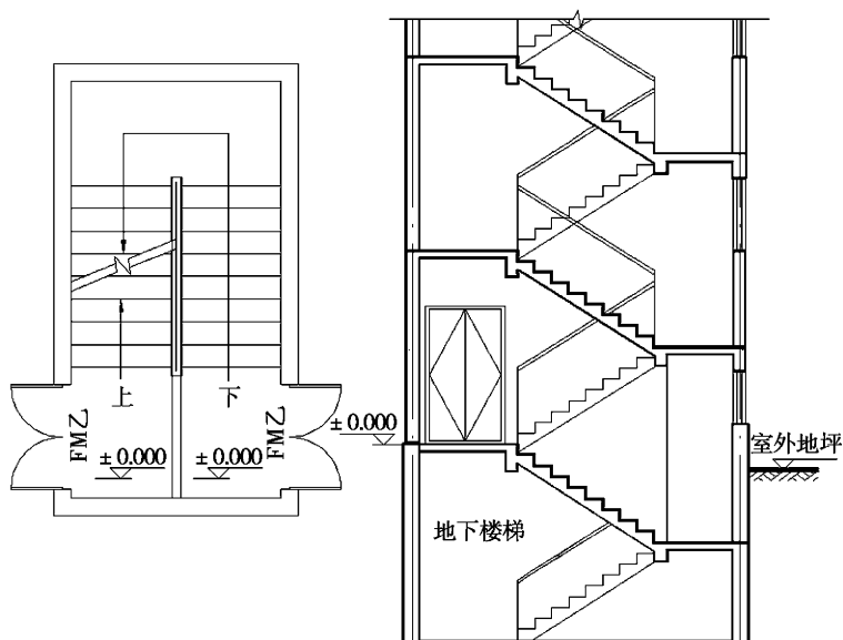
图3 地上和地下楼梯间“不共用”示意图
