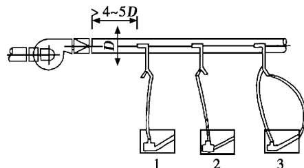
1 - 全正压;2 - 静正压;3 - 动压
