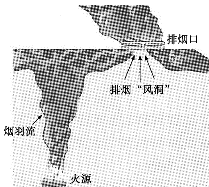
图 18 排烟口的最高临界排烟量示意图
