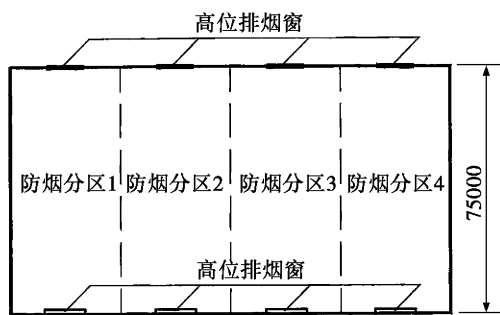
图8 具备对流条件场所自然排烟窗的布置
