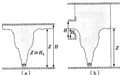
图 11 最小清晰高度示意图
