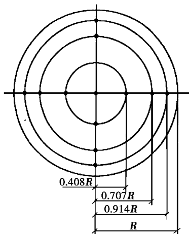
图 22 圆形风管测点布置图
