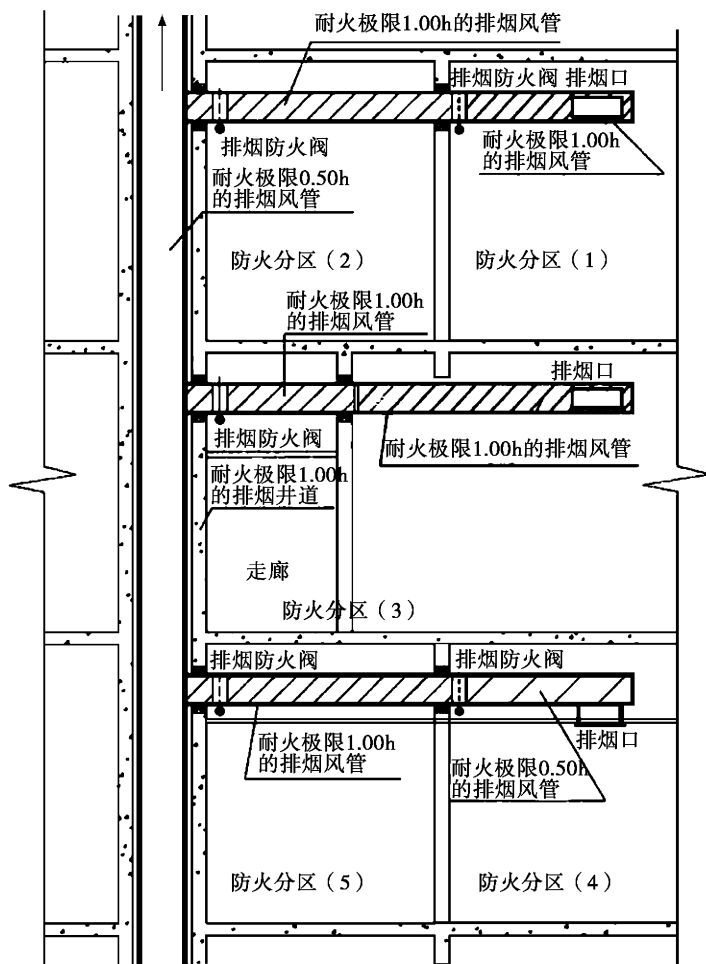
图 20 排烟管道布置示意图
