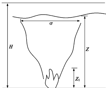
图 13 轴对称型烟羽流
