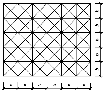
图 21 矩形风管测点布置图
