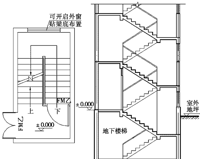
图 2 地上和地下楼梯间“共用”示意图
