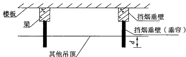
图 7 开孔率小于等于 25% 或开孔不均匀的通透式吊顶及一般吊顶
