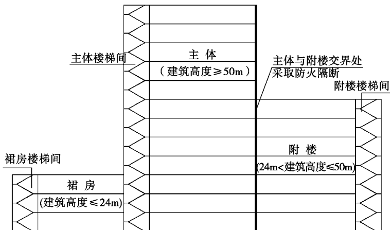
图 1 主体、裙房和附楼示意图
