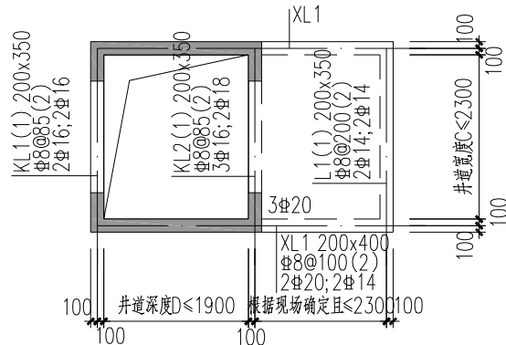
二~九层结构布置图
