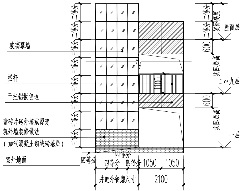
立面样式四幕墙分隔图 (干挂铝板和玻璃幕墙)
