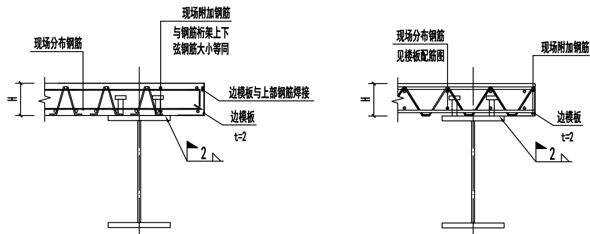
板边做法一
