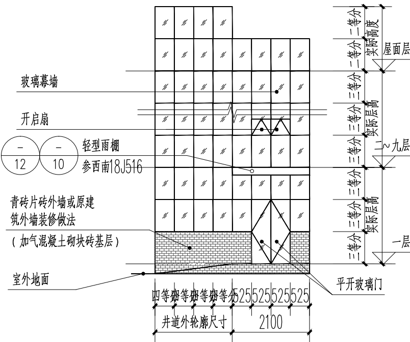
立面样式三幕墙分隔图 (玻璃幕墙)
