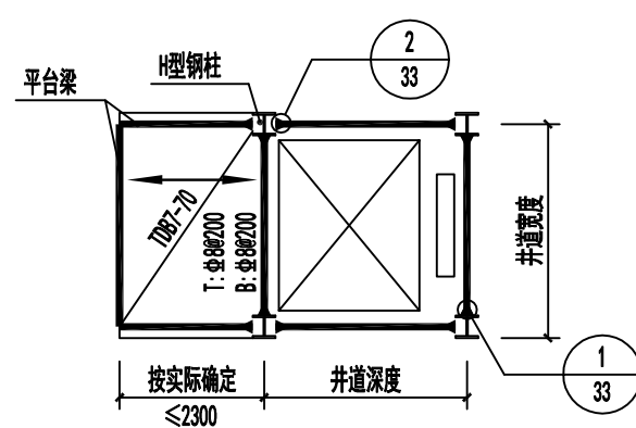
1-1 (H型钢柱标准层平面示意)
