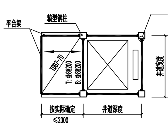
1-1 (箱型钢柱标准层平面示意)
