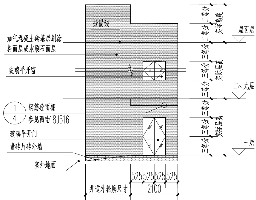
立面样式二幕墙分隔图
