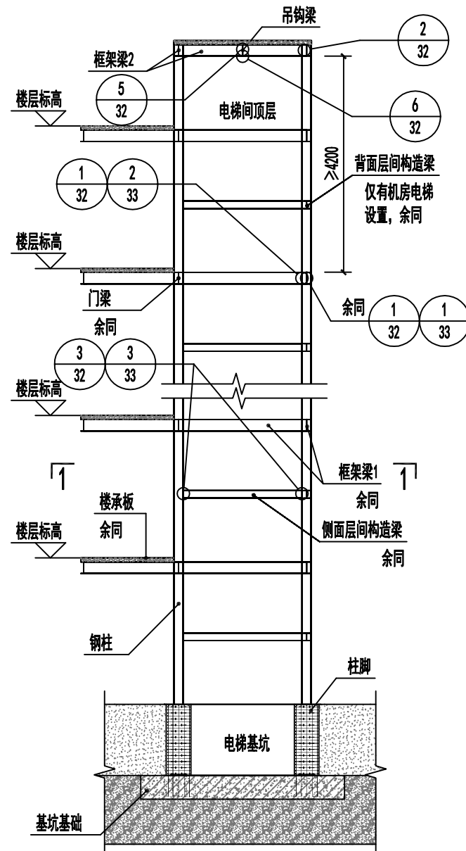
电梯井道钢框架剖面图
