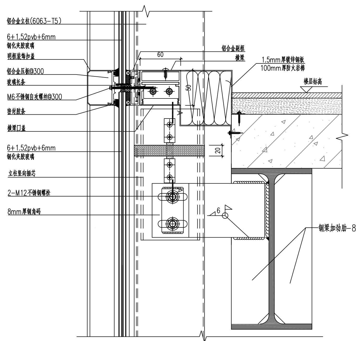
明框玻璃幕墙楼层标高竖向节点（钢结构）
