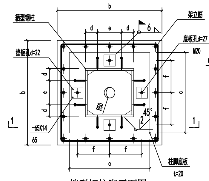
箱型钢柱脚平面图
