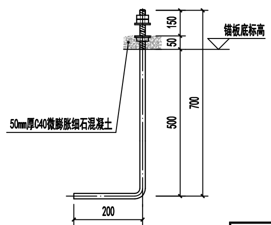
M20柱脚锚栓大样 材质Q235B
