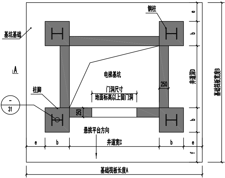
基坑基础大样
