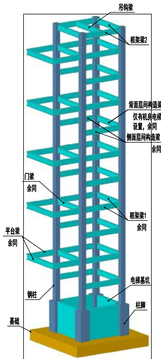
电梯井道钢框架轴测图
