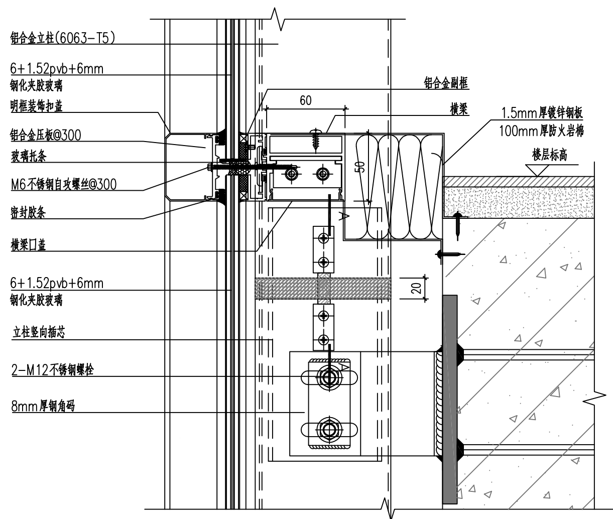
明框玻璃幕墙楼层标高竖向节点（混凝土结构）
