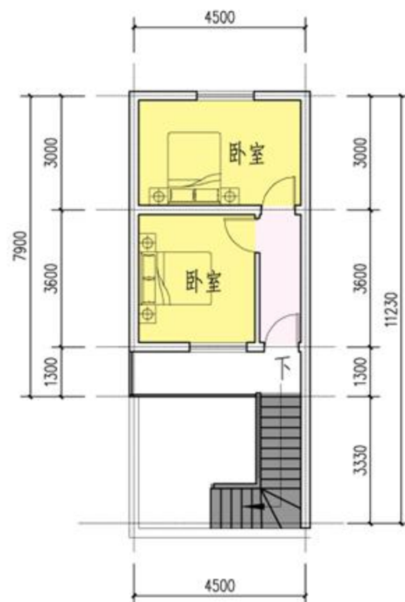
危房改造 (二) 二层平面图 1:100
