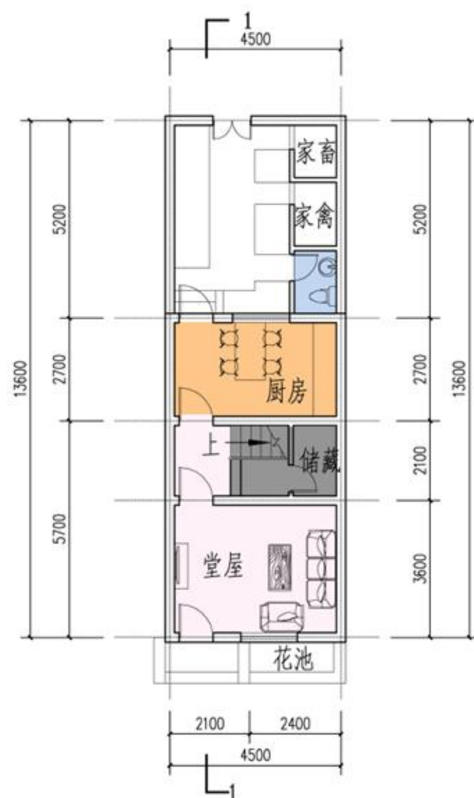
危房改造 (一) 一层平面图 1:100
