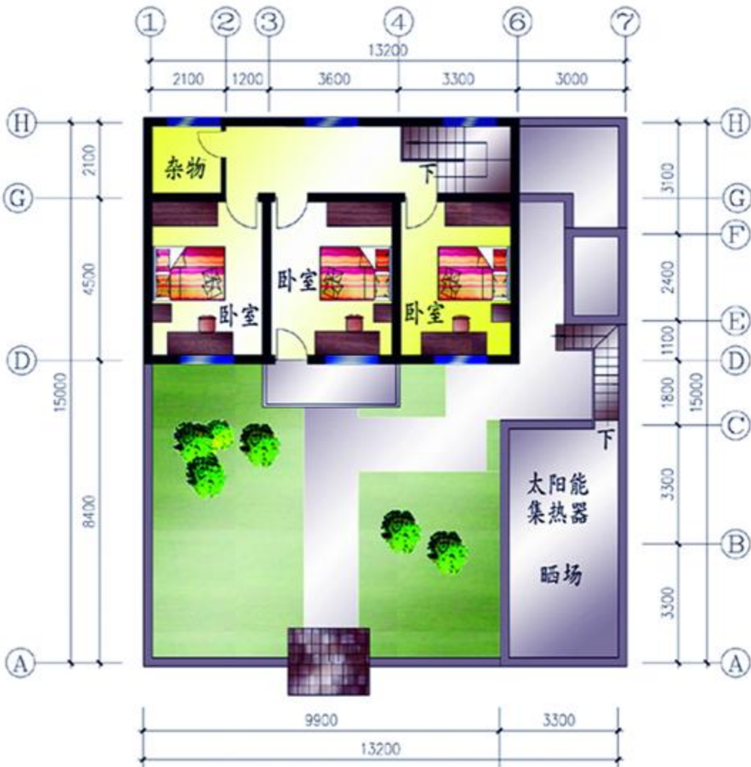
二层平面图
