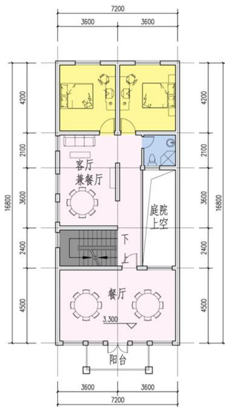
农家乐二层平面图 1:100
