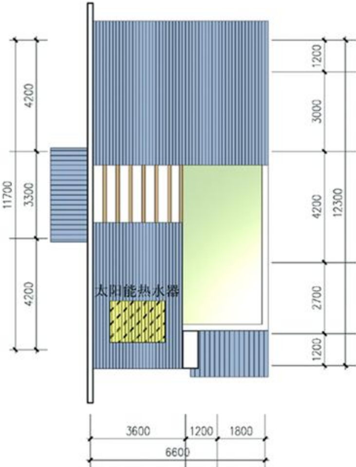
屋顶平面图
