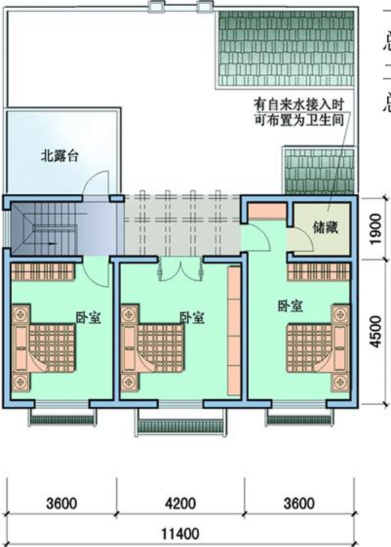
二层平面
