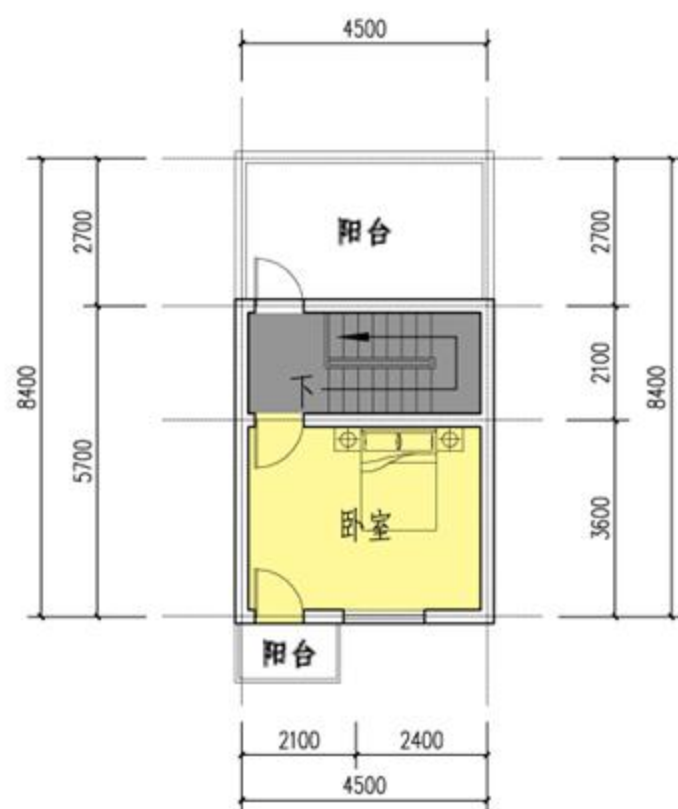
危房改造 (一) 二层平面图 1:100
