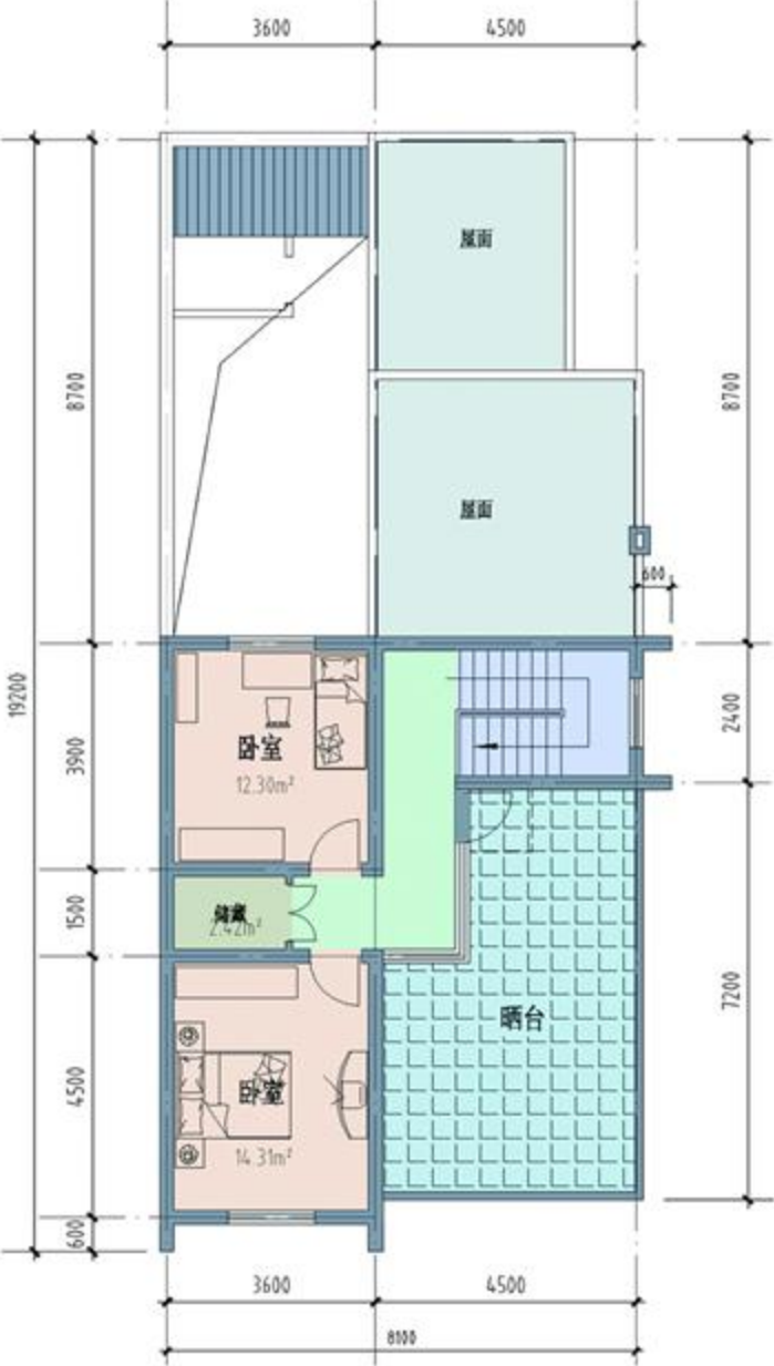
二层平面图
