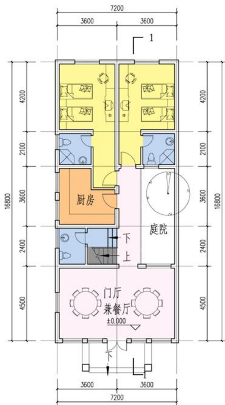
农家乐一层平面图 1:100
