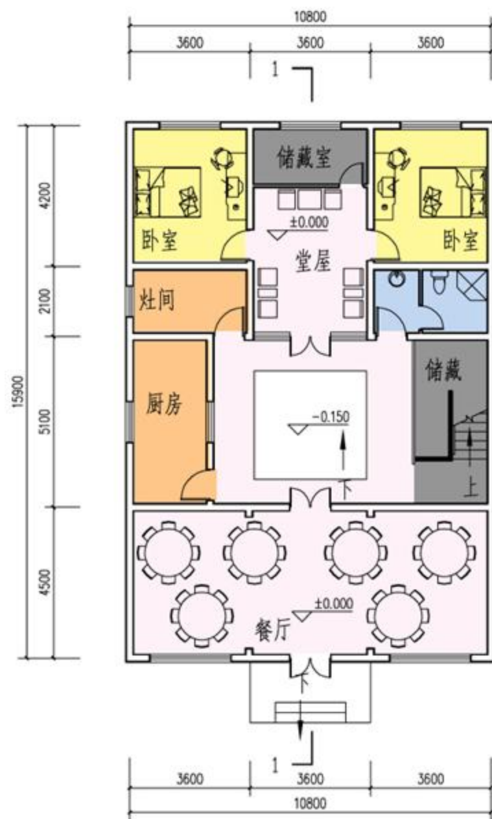
一层平面图 1:100
