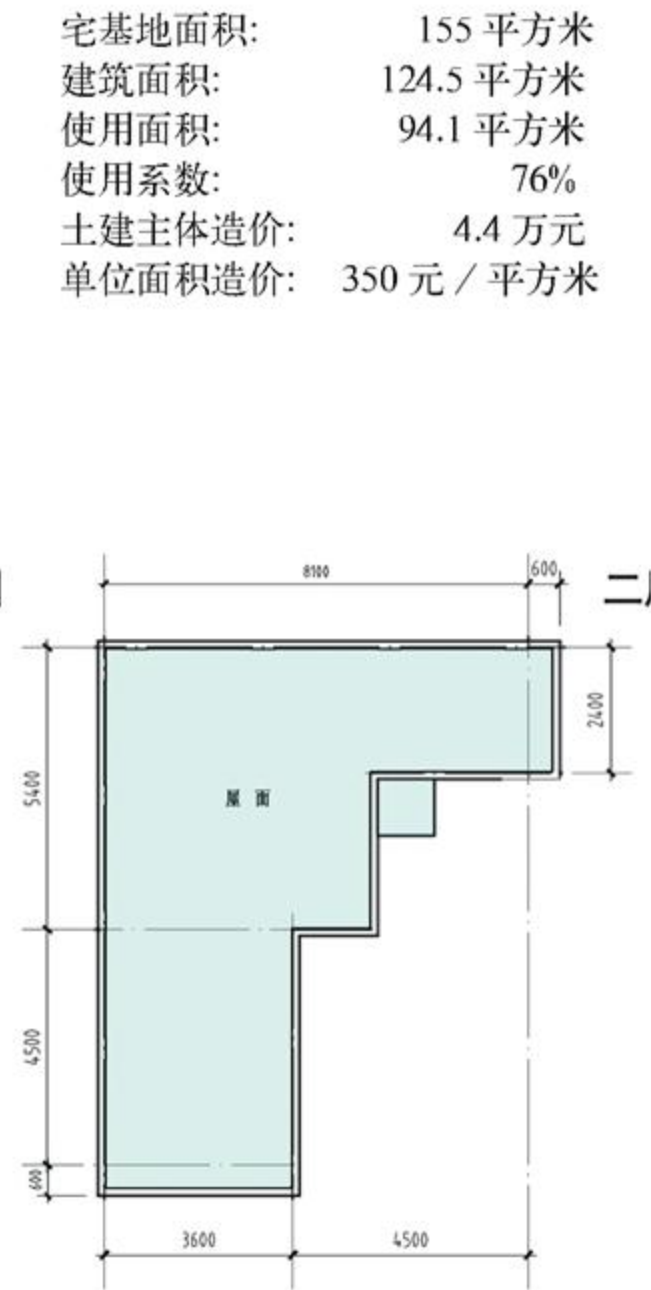
屋顶平面图
