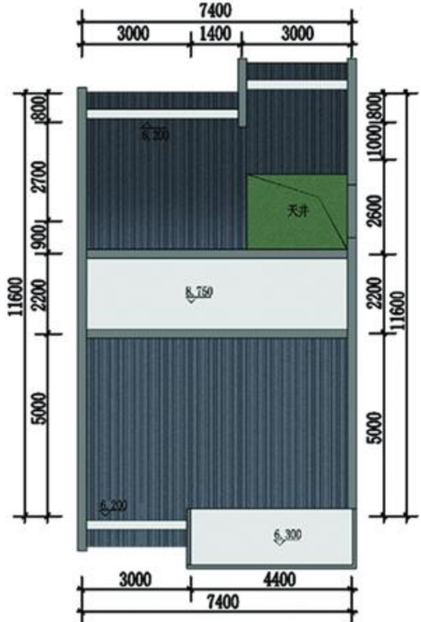
三层平面图
