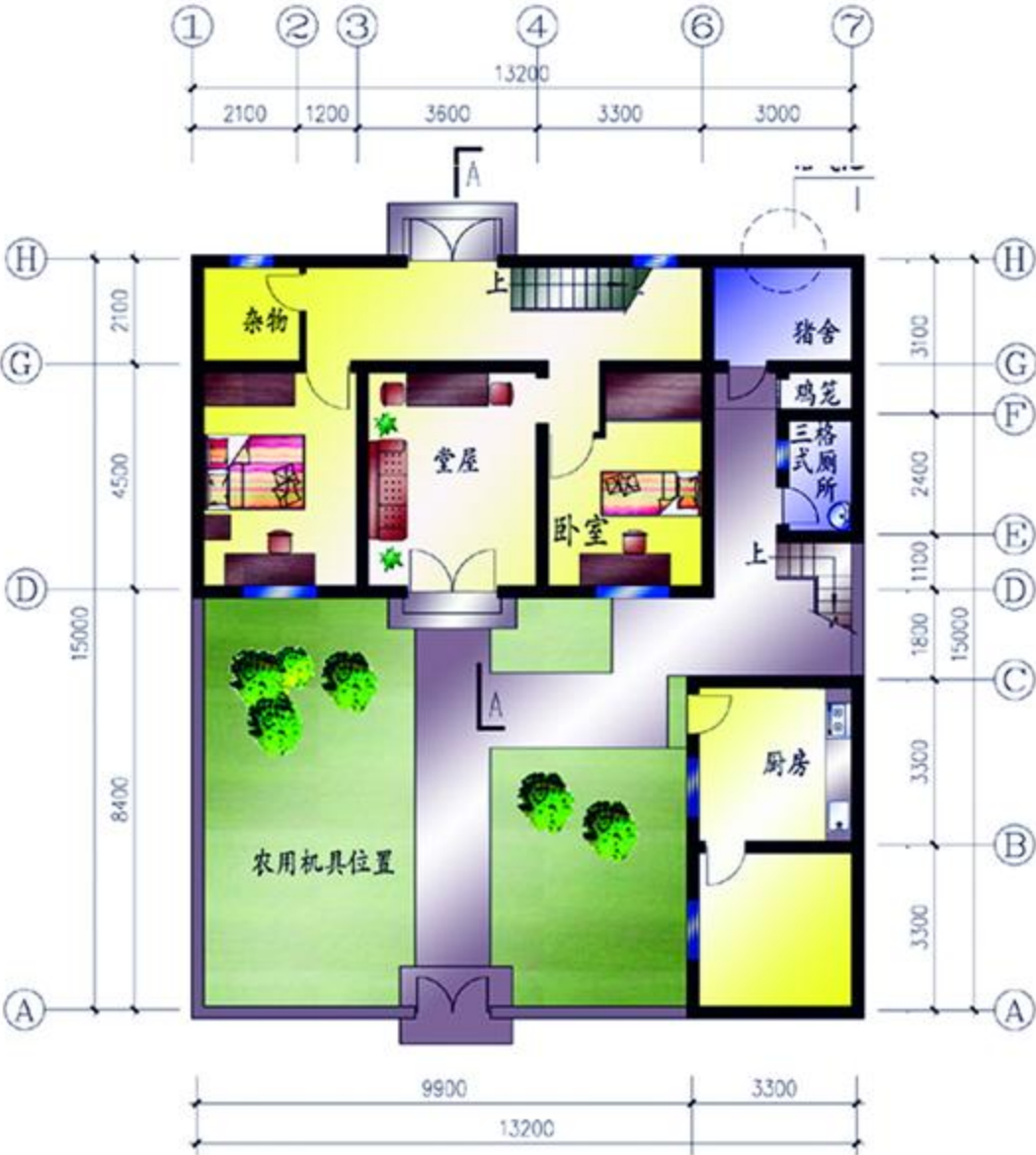
底层平面图
