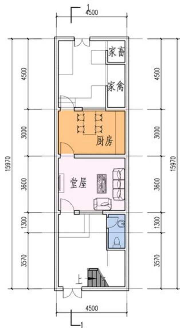
危房改造 (二) 一层平面图 1:100
