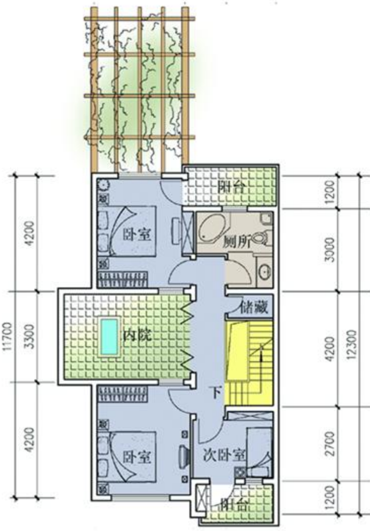
二层平面图
