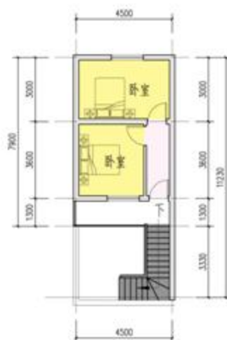
危房改造(二)二层平面图 1:100 32m 2
