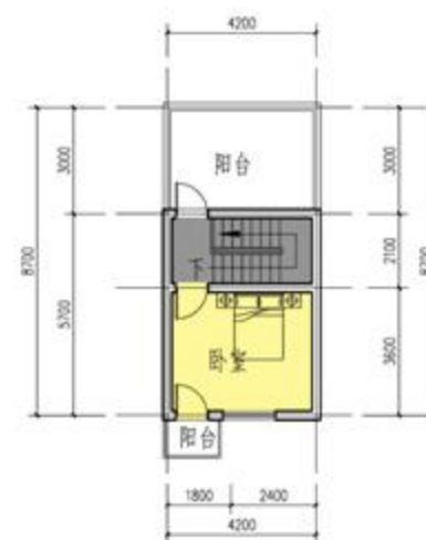
危房改造(一)二层平面图 1:100 26m 2
