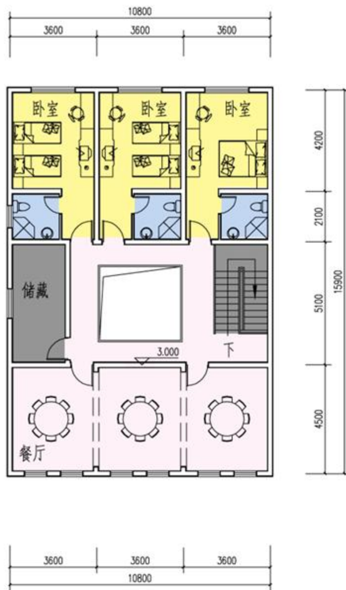
二层平面图 1:100
