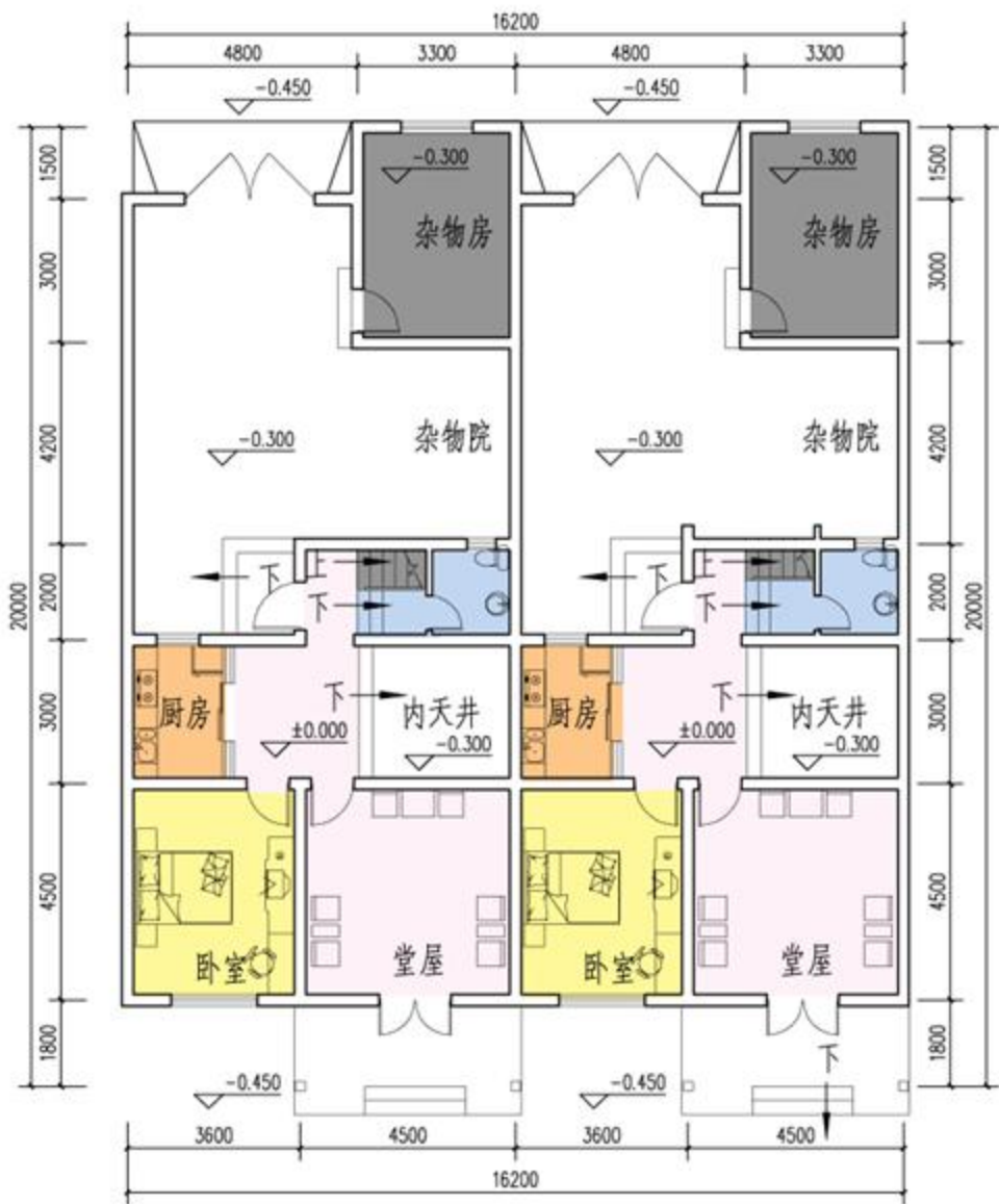
一层平面图 1:100
