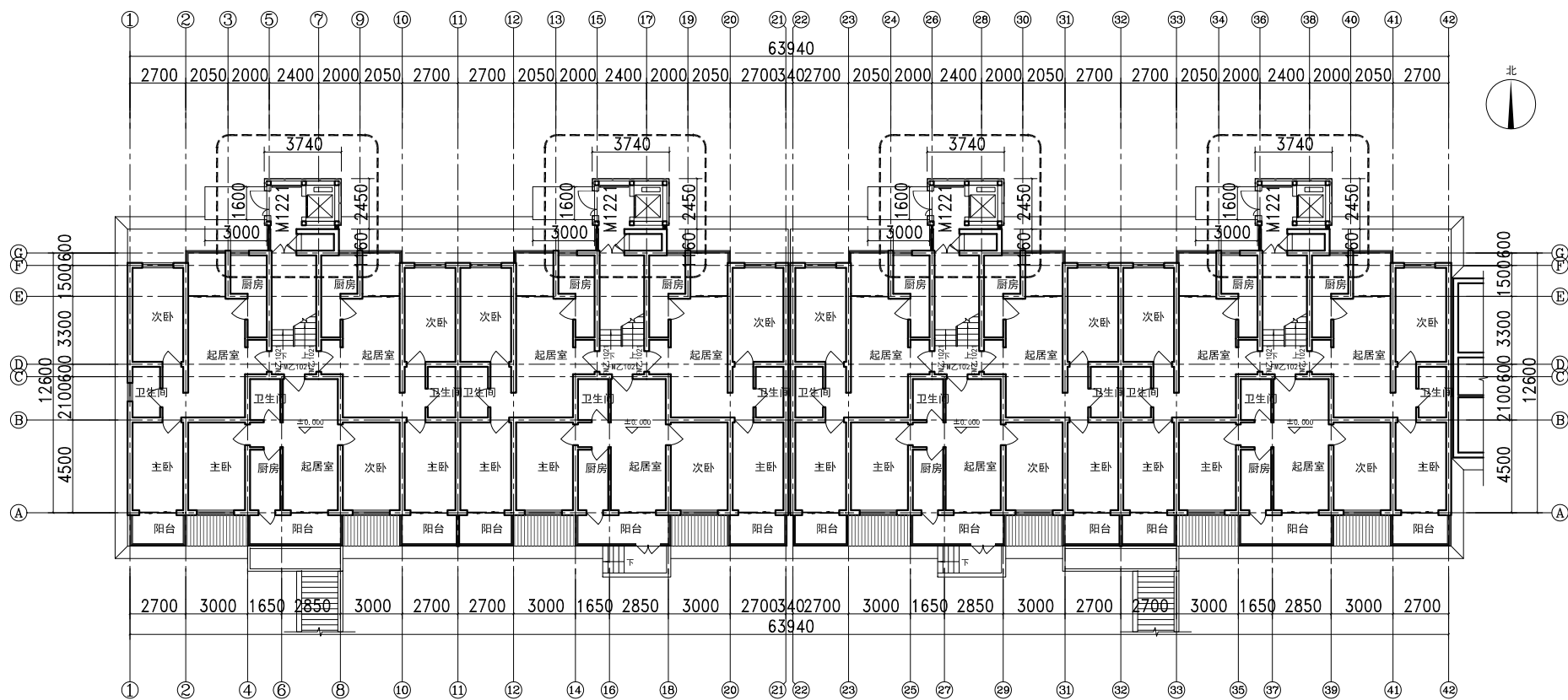
首层平面图
