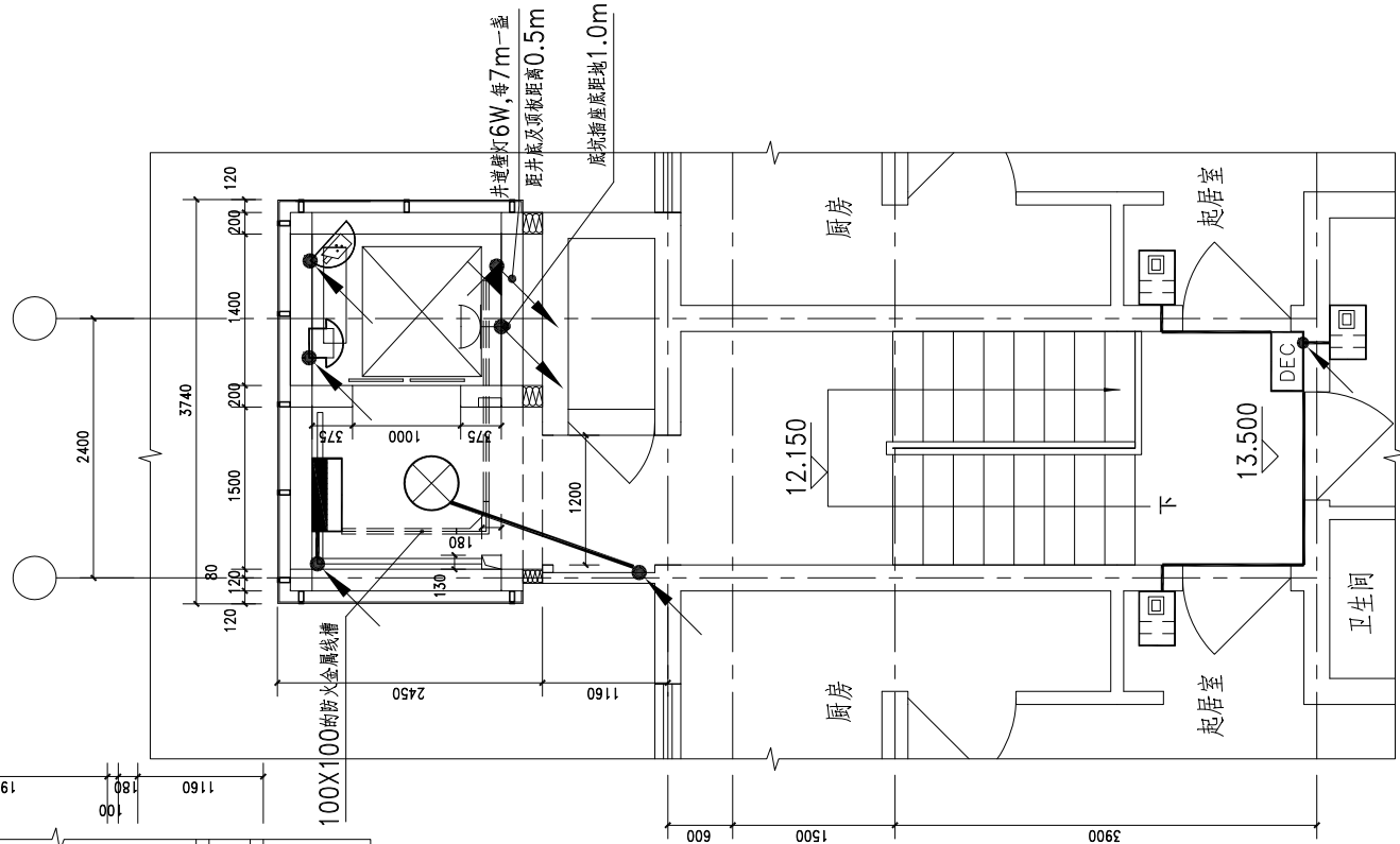
顶层楼道电气平面图
