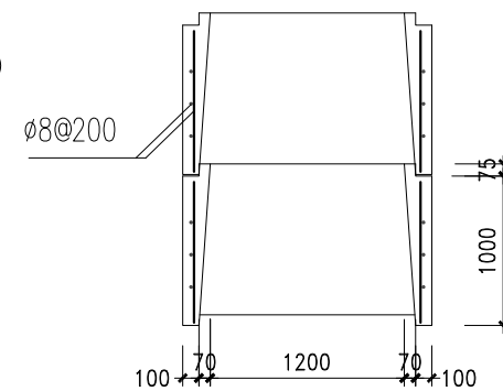
混凝土护壁配筋
