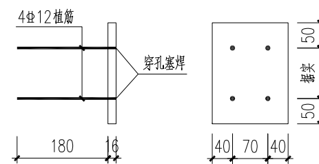
埋件详图
