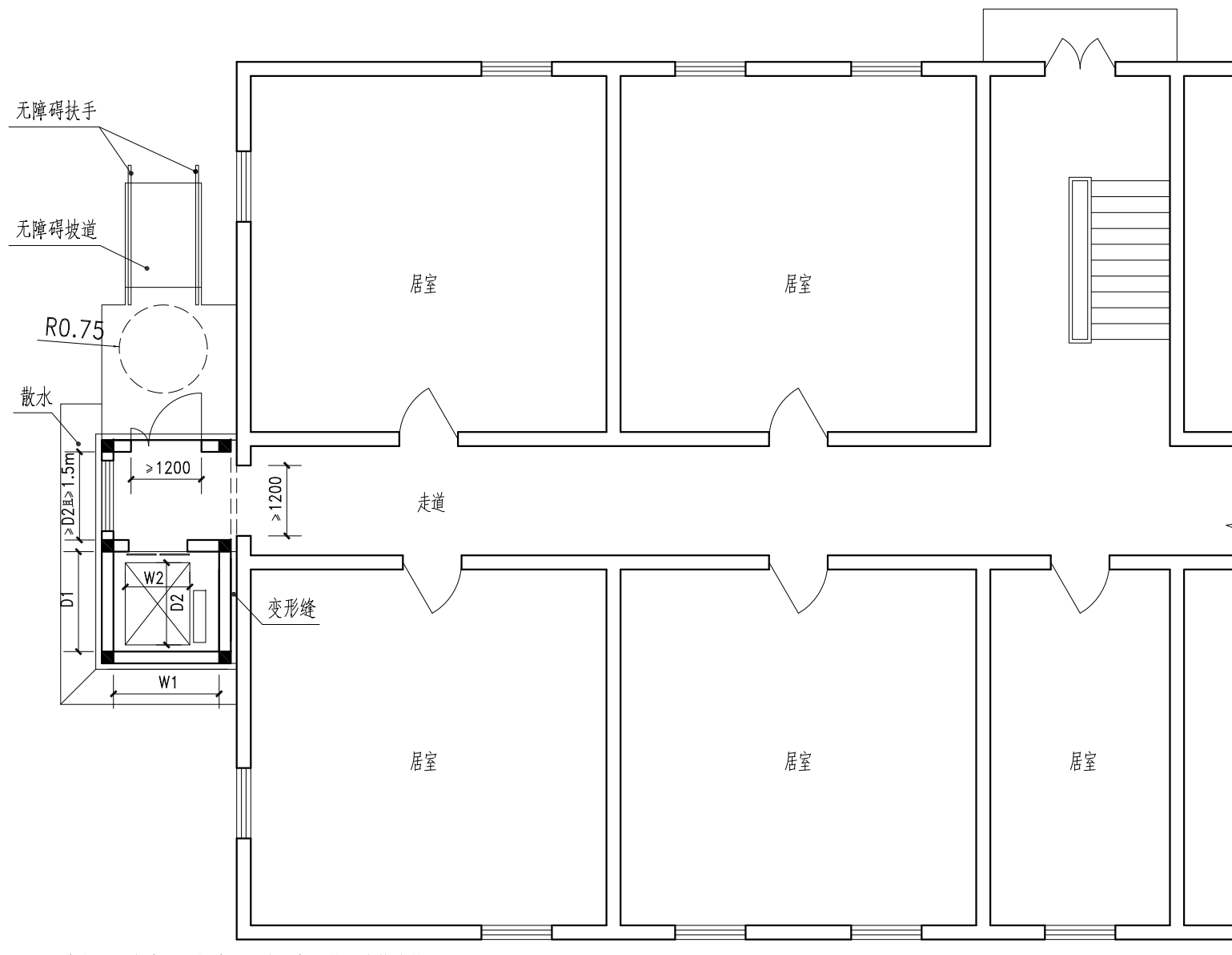
首层平面图
