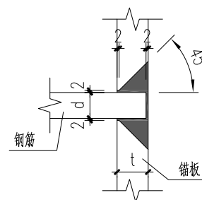
穿孔塞焊构造
