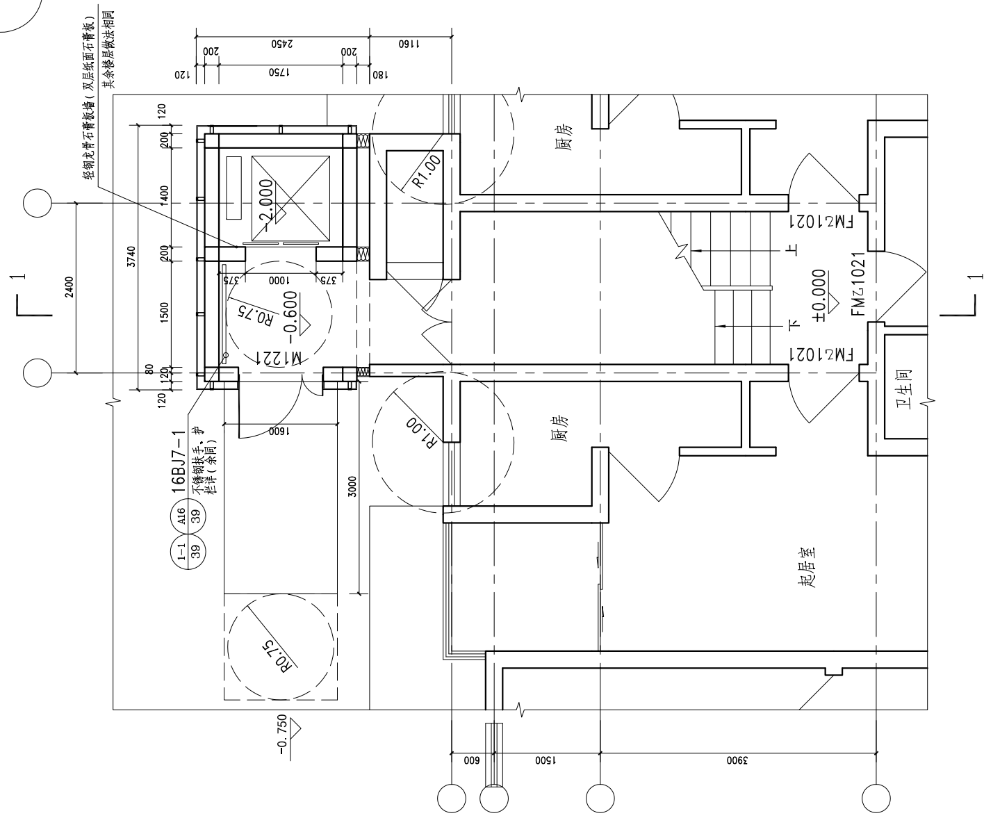
首层平面图
