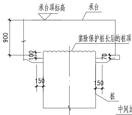
桩头处做法
