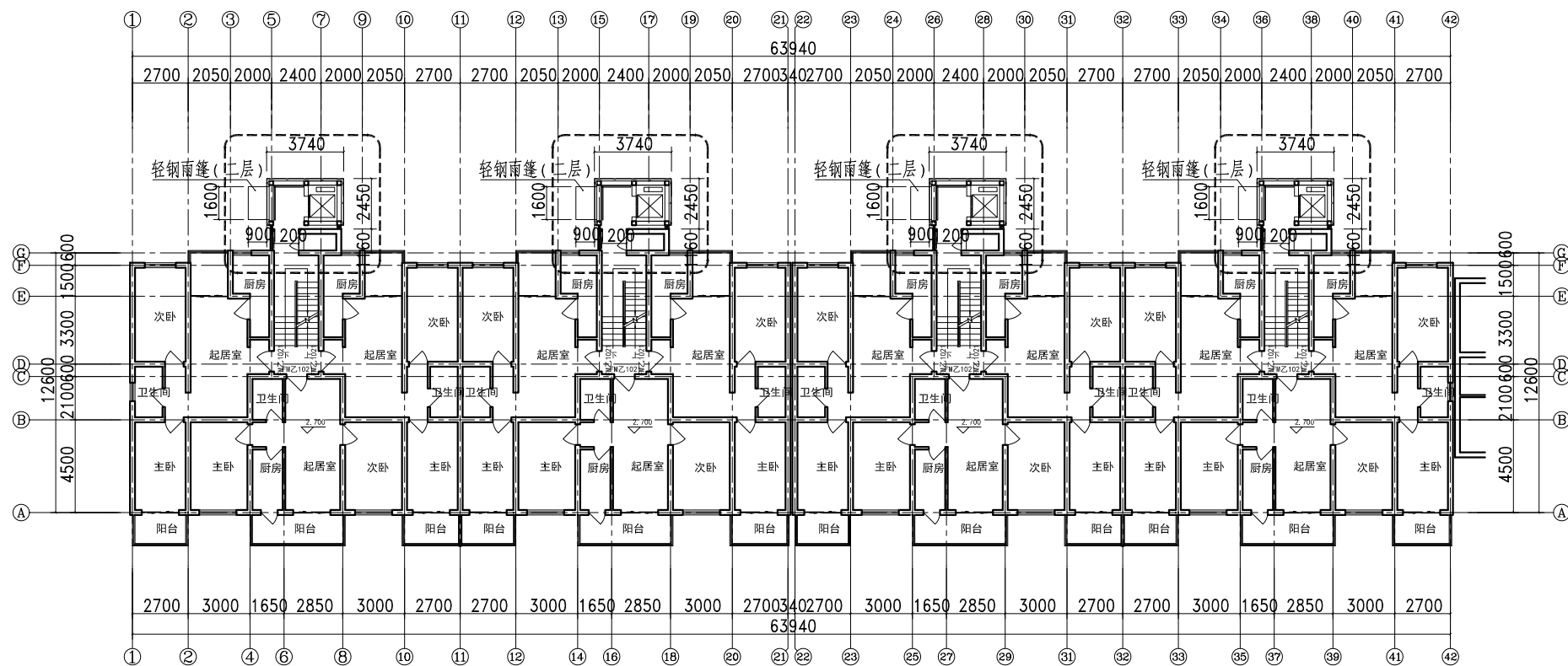
二层平面图
