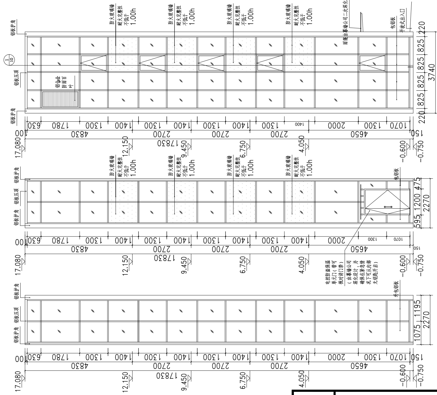
东立面图
