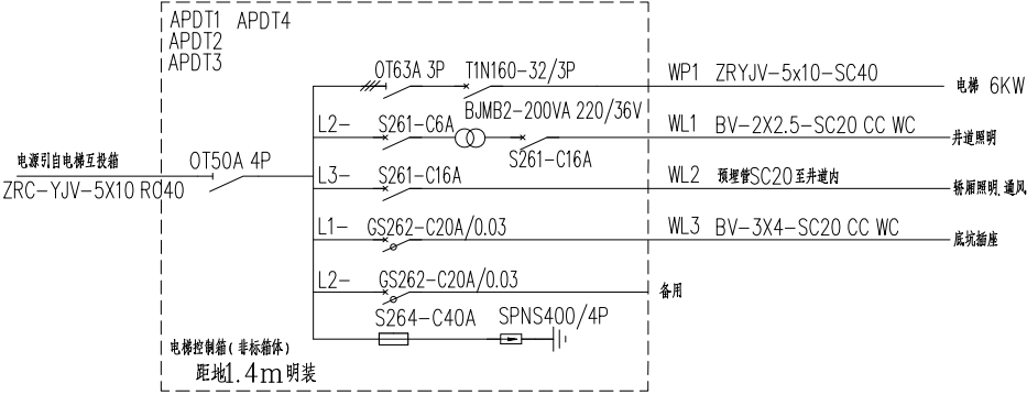
配电系统图
