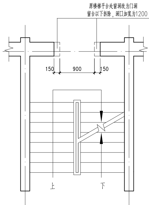
洞口改造示意图
