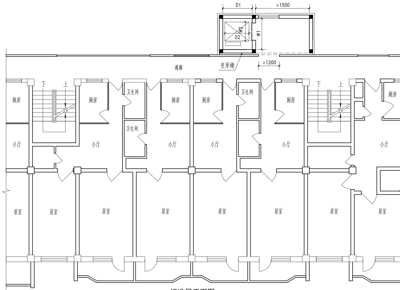
标准层平面图
