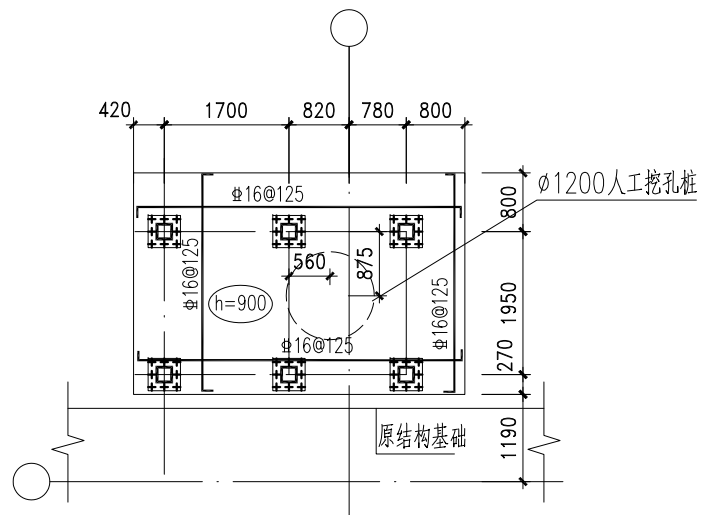
基础平面图
