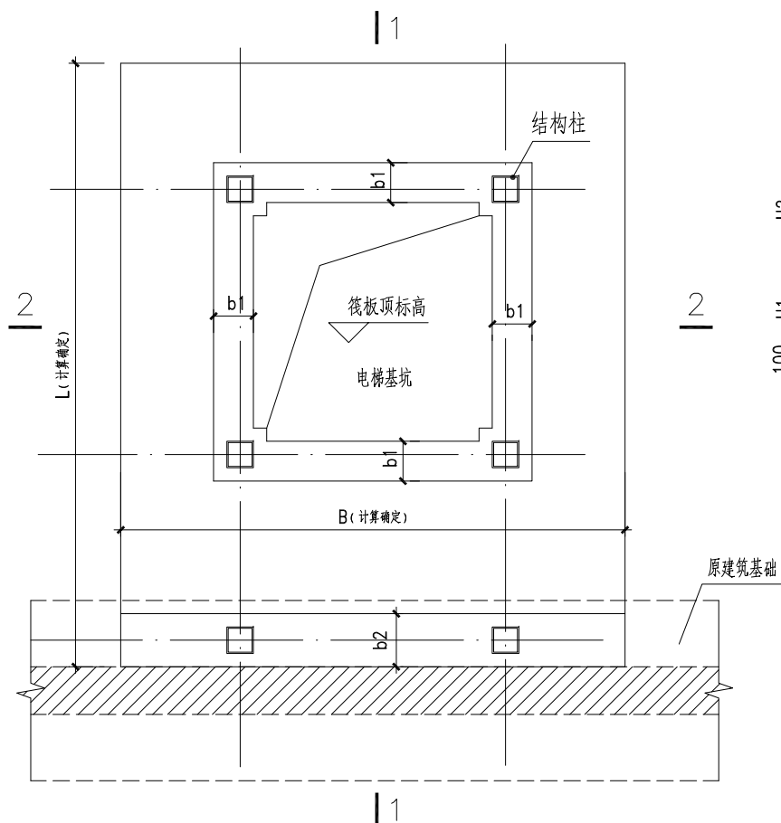
筏板基础平面示意图
