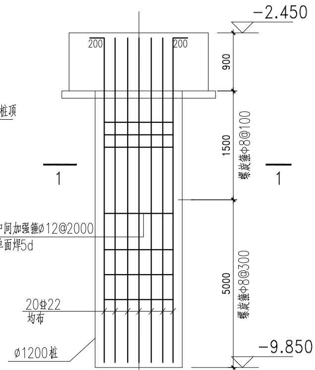
桩配筋图
